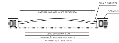
Corte transversal da rua
