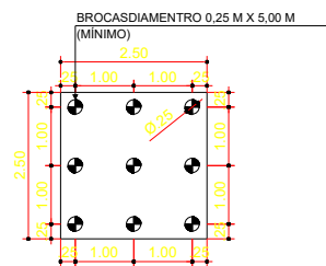
BROCAS VISTA SUPERIOR
