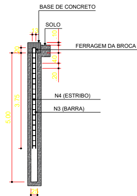
DETALHE DAS BROCAS COM A FERRAGEM
