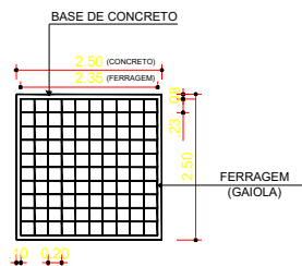
ARMADURA DA BASE VISTA SUPERIOR
