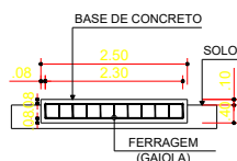
FERRAGEM (GAIOLA) DA BASE VISTA DE LADO
