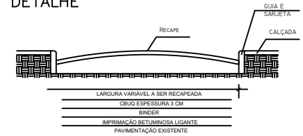
Corte transversal da rua sem escala
