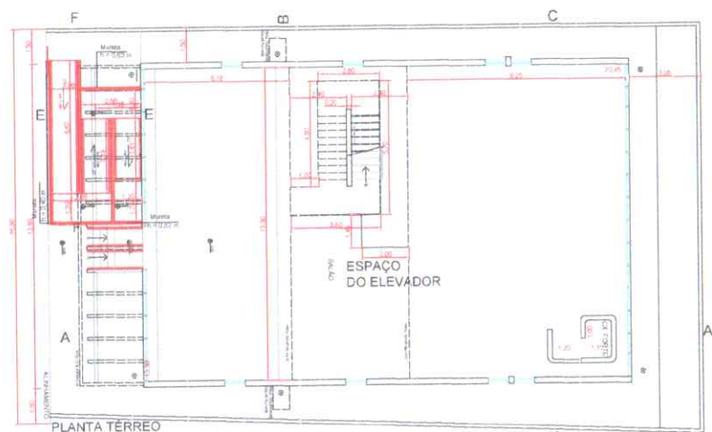
PLANTA TÉRREO ESC. 1:100
