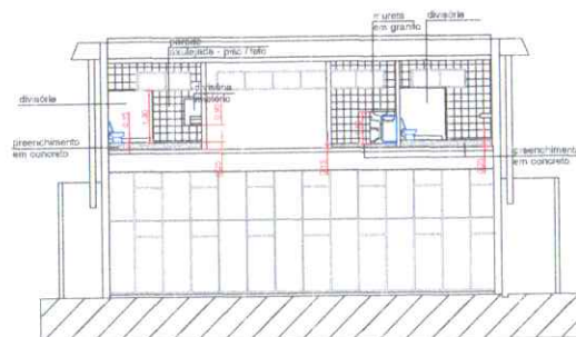
CORTE CC ESC. 1:100
