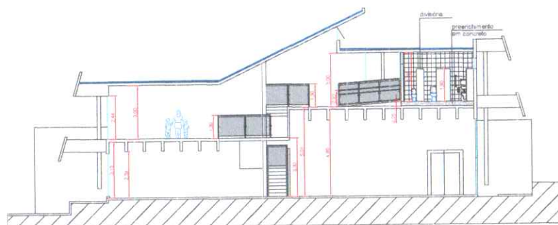
CORTE AA ESC. 1:100
