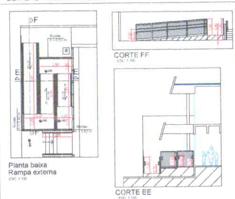
DETALHE - RAMPA EXTERNA
