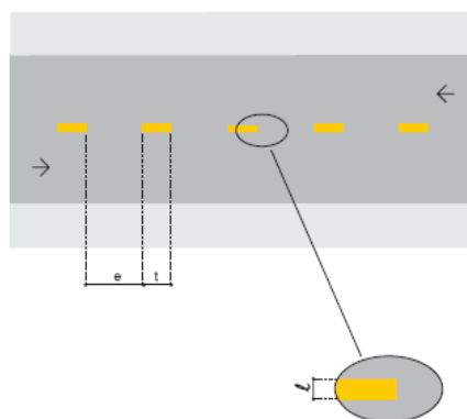
Linha simples seccionada (LFO-2)
