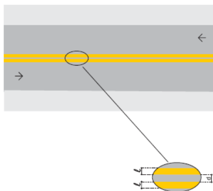
Linha dupla contínua (LFO-3)
