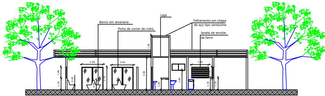
Corte AA Esc.: 1:100
