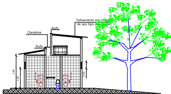
Corte BB Esc.: 1:100
